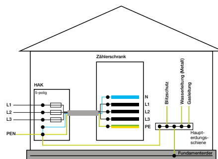
TN-System
