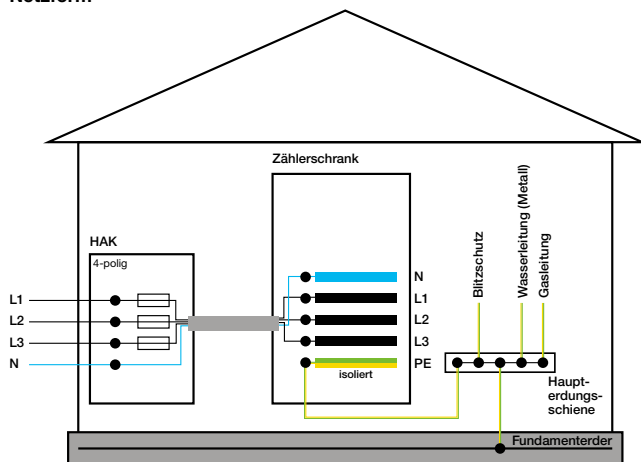
TT-System
