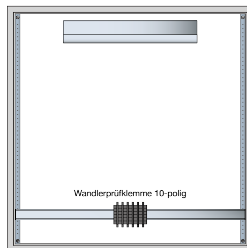
Beistellung der Zählerwechselplatte muss bauseits erfolgen
