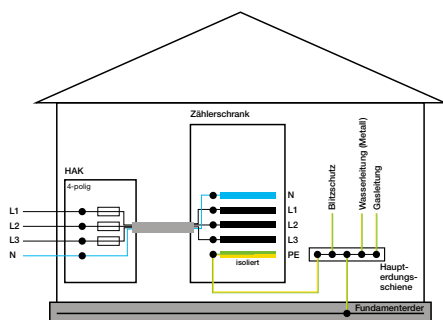
TT-System
