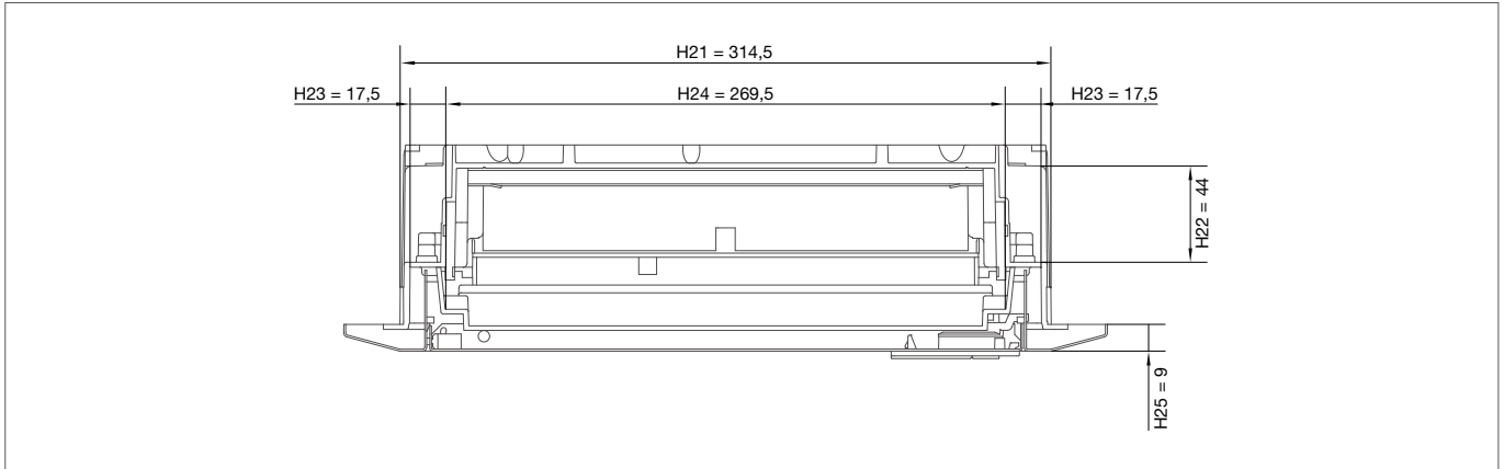
Draufsicht VU36
