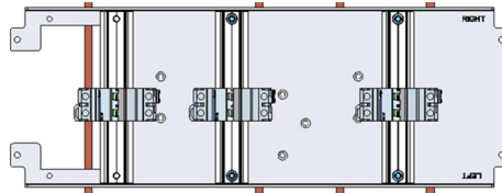
DIN Schiene vertikal (1 bis max 3) für Reiheneinbaugeräte
