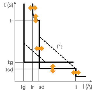
Auslösecharakteristik - L SIG
