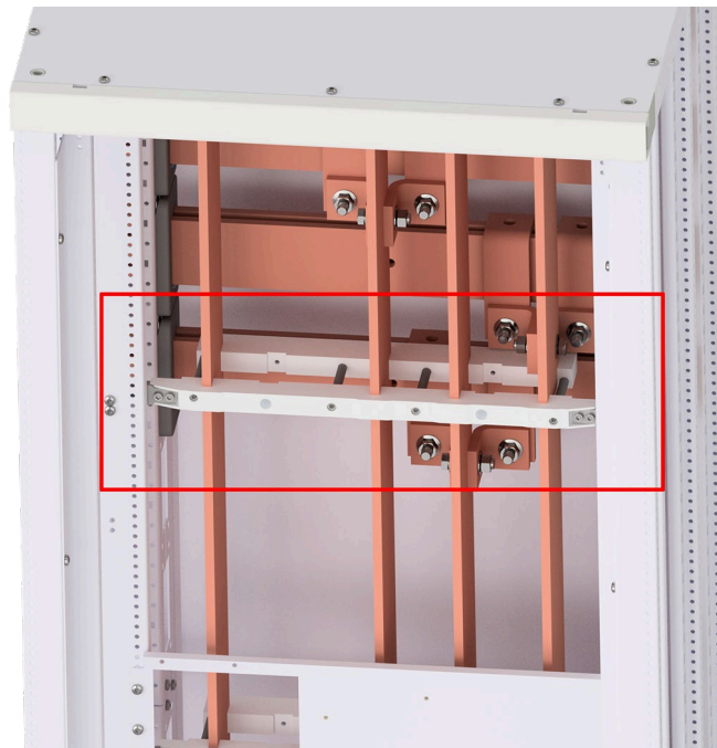
Einbaubeispiel Feld-Sammelschienenenträger U-SST...
