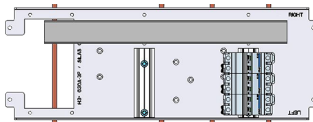
DIN Schiene vertikal (1 bis max 2) mit Kabelkanal
