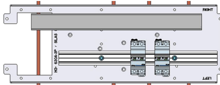
DIN Schiene horizontal unten mit Kabelkanal
