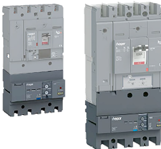
FI-Block (RCD-Block), Beispiele
