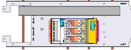
SILAS Gr. 00 (160 A) mit Kabelkanal
