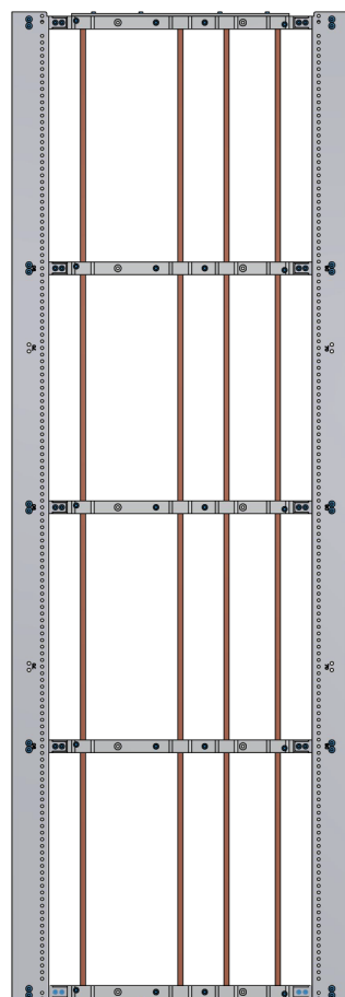
Oberer F-SaS Träger mit Isolierplatte
