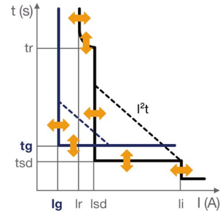
Auslösecharakteristik - Energy
