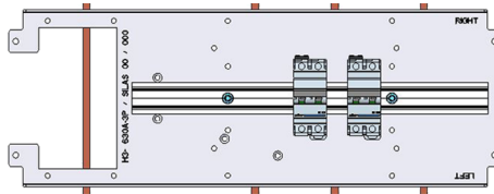
DIN Schiene horizontal mitte
