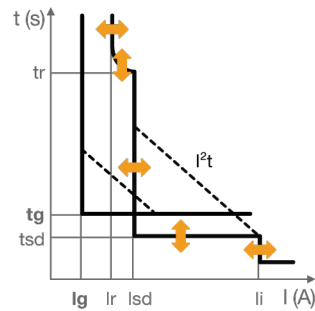
Auslösecharakteristik - LSI
