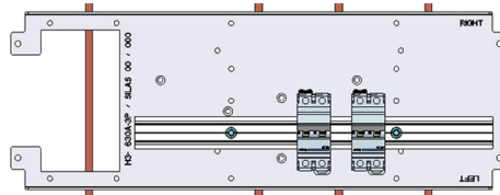
DIN Schiene horizontal unten
