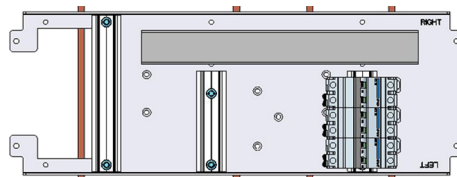
DIN Schiene vertikal (1 bis max 3) mit Kabelkanal
