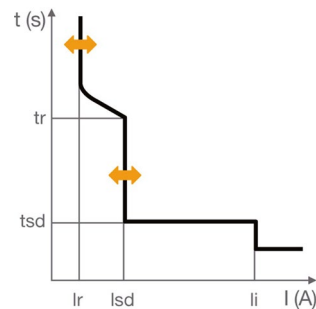
Auslösecharakteristik - LSnl
