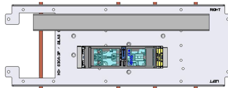
SILAS Gr. 000 (100 A) mit Kabelkanal
