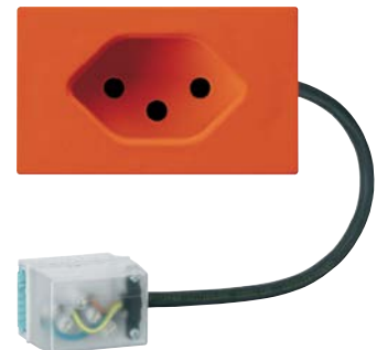
FLF Typ 13 L1 Orange mit Power Anschlussdose Best.-Nr.: WH37682406D, E-Nr.: 663 214 163
