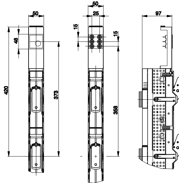
Messgerätehalter lang
