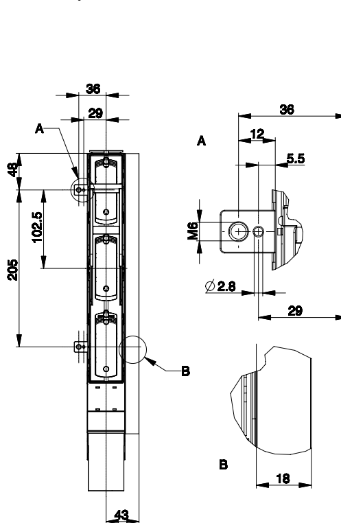
Abstützclip und Profilblende
