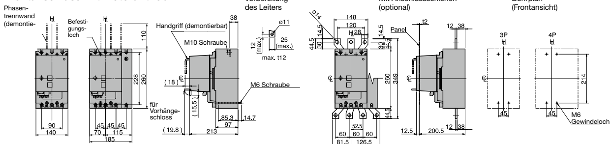
Vorbereitung des Leiters
