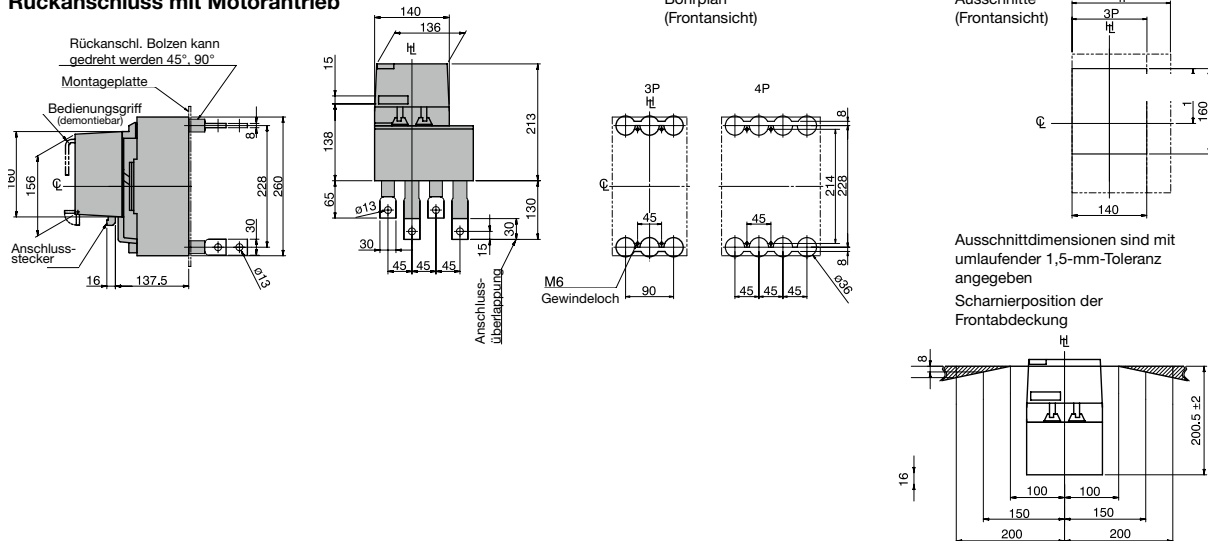
Bohrplan (Frontansicht)
