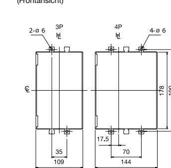
Bohrplan (Frontansicht)
