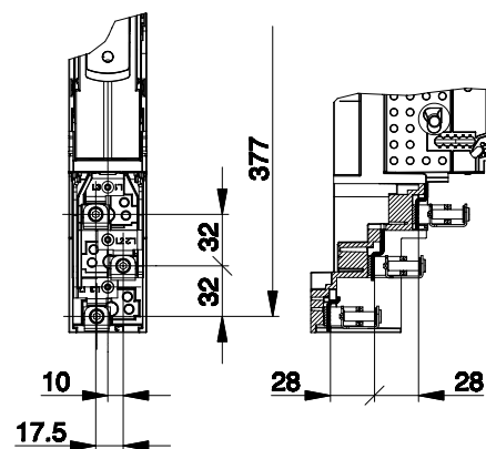
Rahmenklemme max. 95 mm 2
