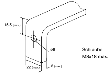
Detail vom Verbindungsstück Angeordnet für Rückanschluss
