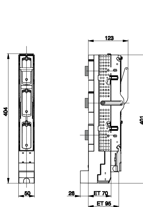
3-polig schaltbar mit kurzer Anschlussraumabdeckung
