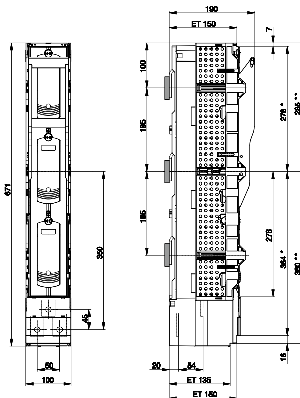
Kurze Anschlussraumabdeckung
