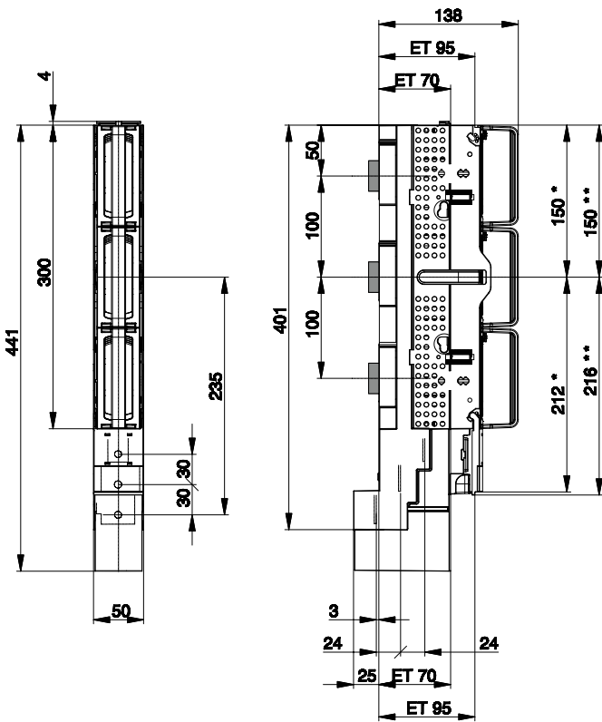
1-polig schaltbar mit Standard-Anschlussraumabdeckung
