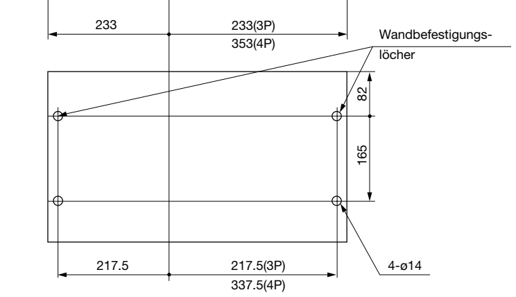
Montagebohrungen
