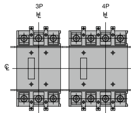
(Rückansicht)
