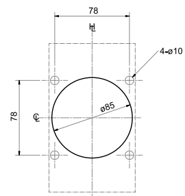
Ausschnitt
