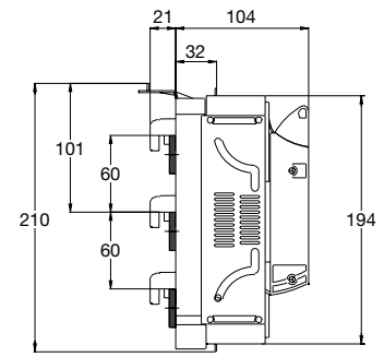
Einbautiefe 32 mm
