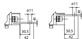
Detail vom Verbindungsstück Angeordnet für Rückanschluss
