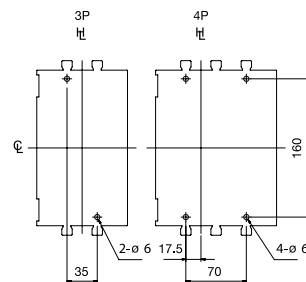
Bohrplan (Frontansicht)
