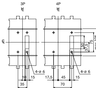
Bohrplan (Frontansicht)
