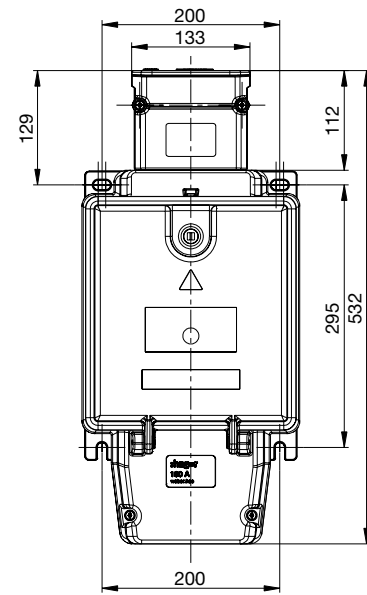
ARE-Modul oben
