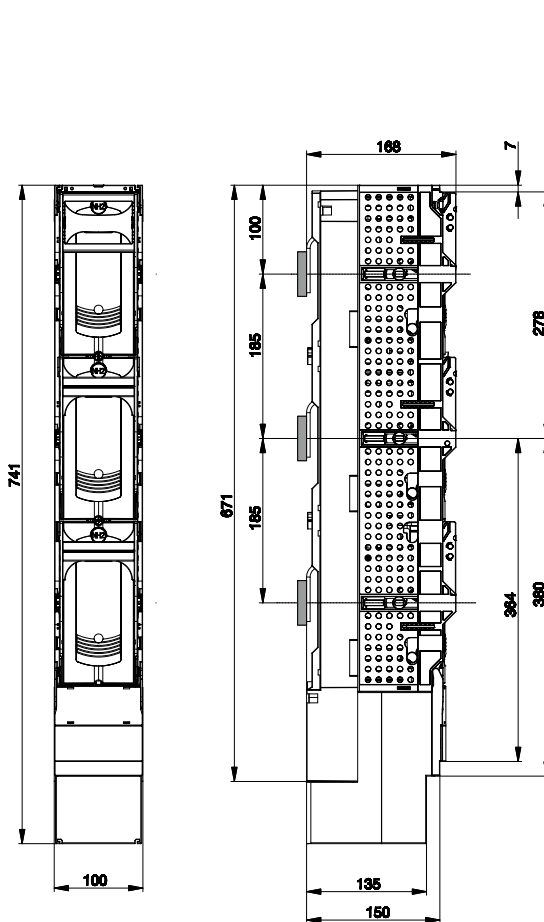
Niedrige Einbautiefe
