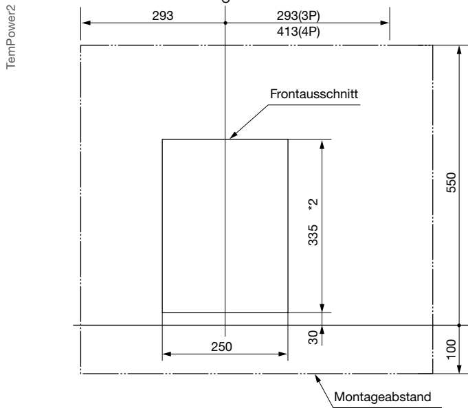
Ausschnitte
