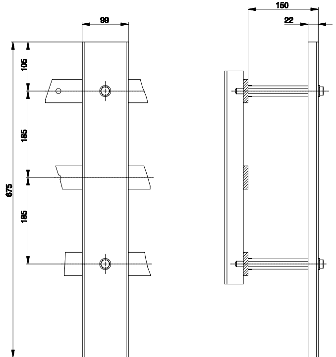
Reserveplatzabdeckung für Einbautiefe 150 mm LVZRA
