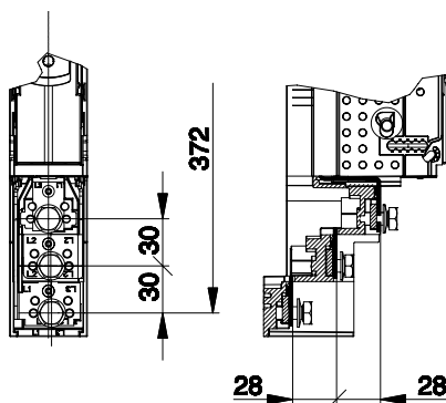
Schraubanschluss M8 x 14
