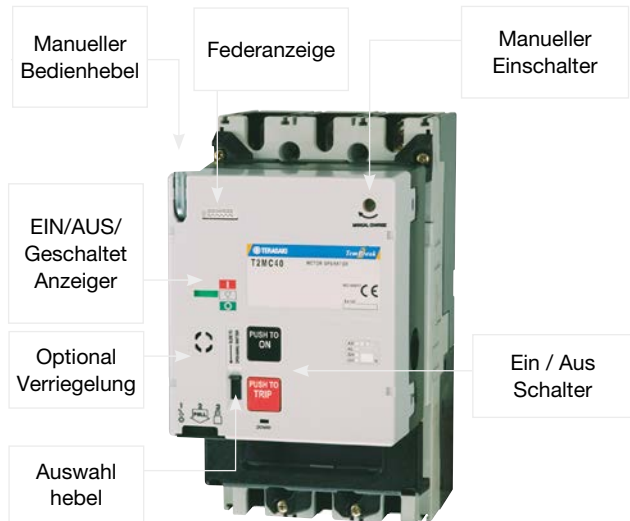
Motorantrieb für 400 A und 630 A Leistungsschalter
