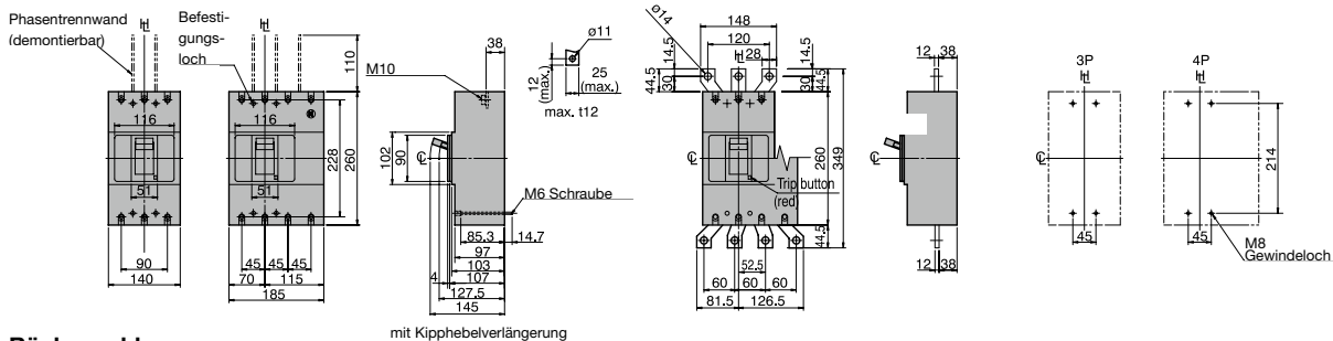
Bohrplan (Frontansicht)
