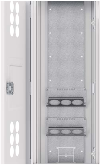
Halterung für Unterputz-Einbaugeräte
