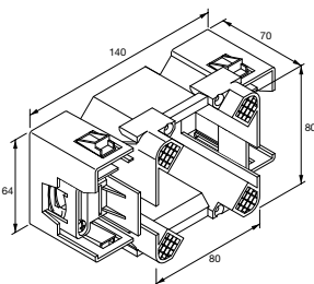
Geräteeinbaudose CEE C-Profil G2744
