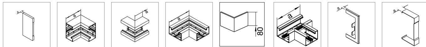
Endplatte PC/ABS halogenfrei Inneneck PVC Ausseneck PVC Flachwinkel PVC Abdeckung für Ausseneck PVC T-Stück PVC Wandanschlussblende Stahlblech Schnittkaskierung Stahlblech
